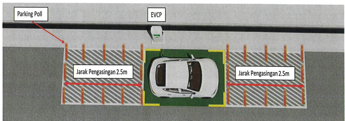
Gambar rajah 5 : Susunan selari (180°)
